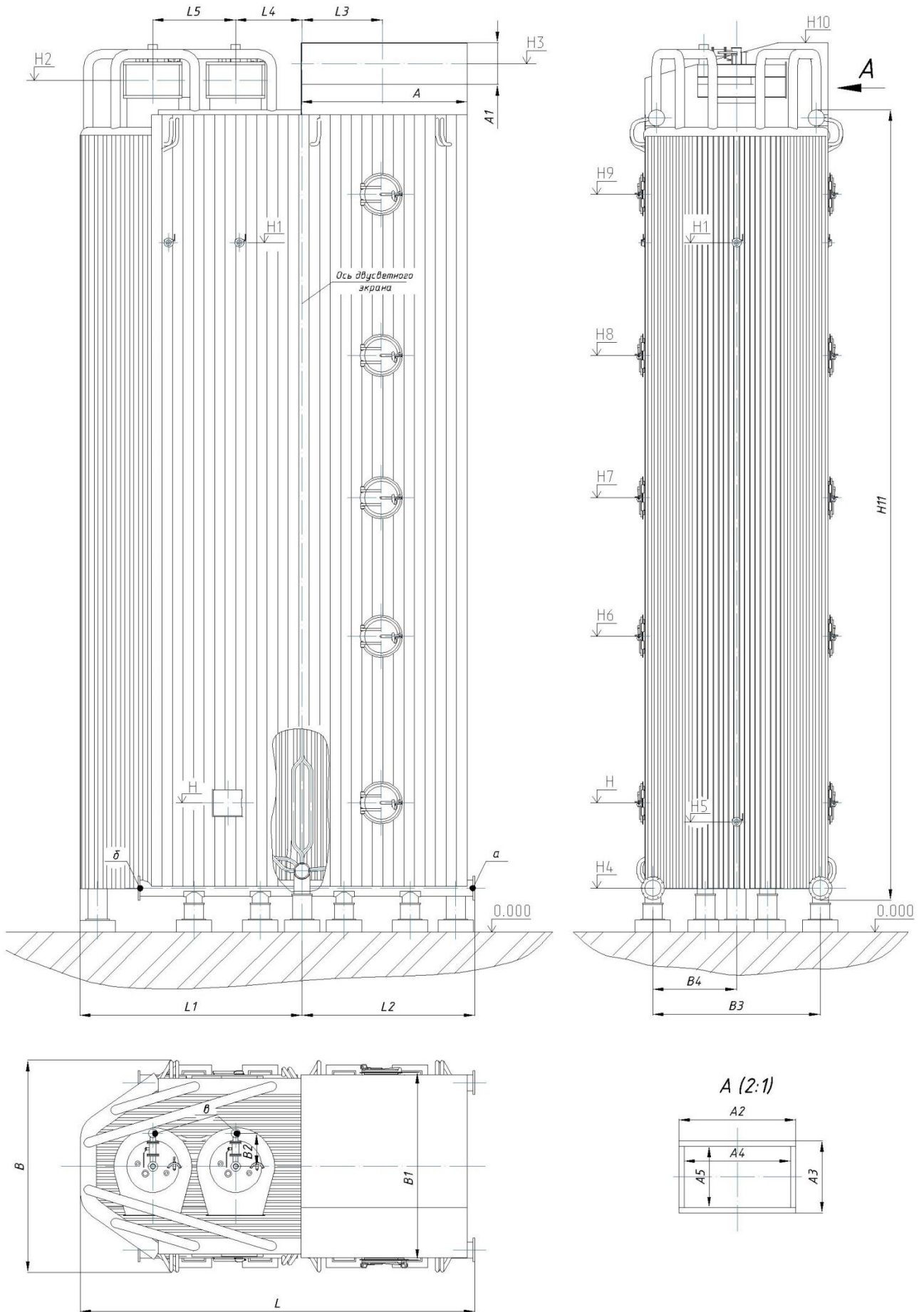
Рисунок 2 – Общие виды котлоагрегата
