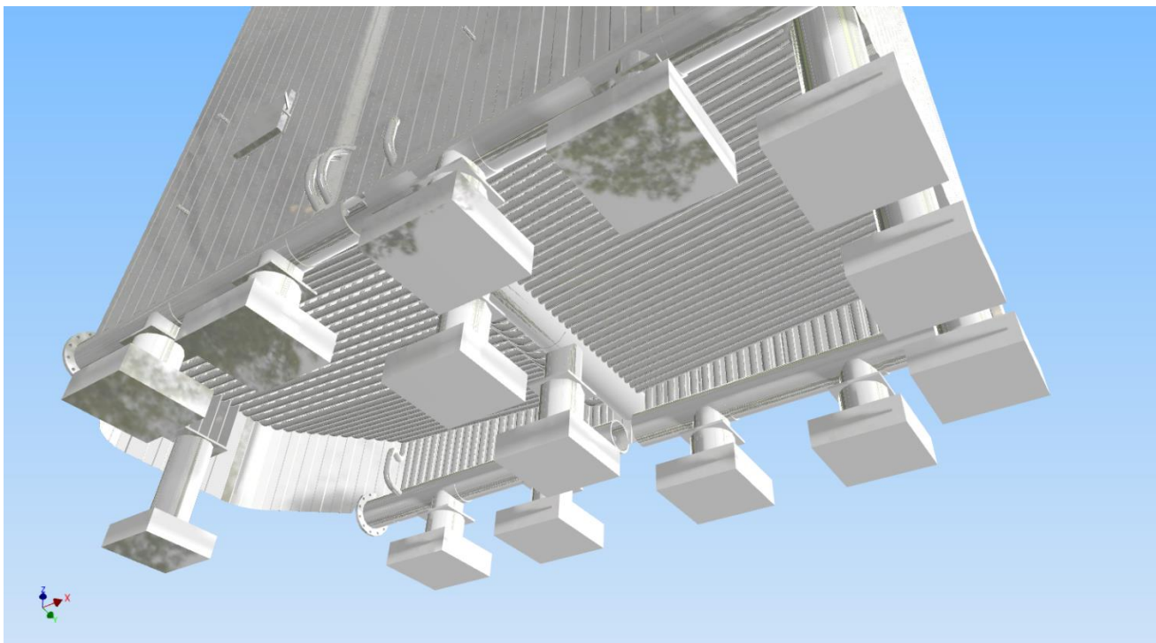
Рисунок 4 – Общий вид котлоагрегата (вид снизу)
