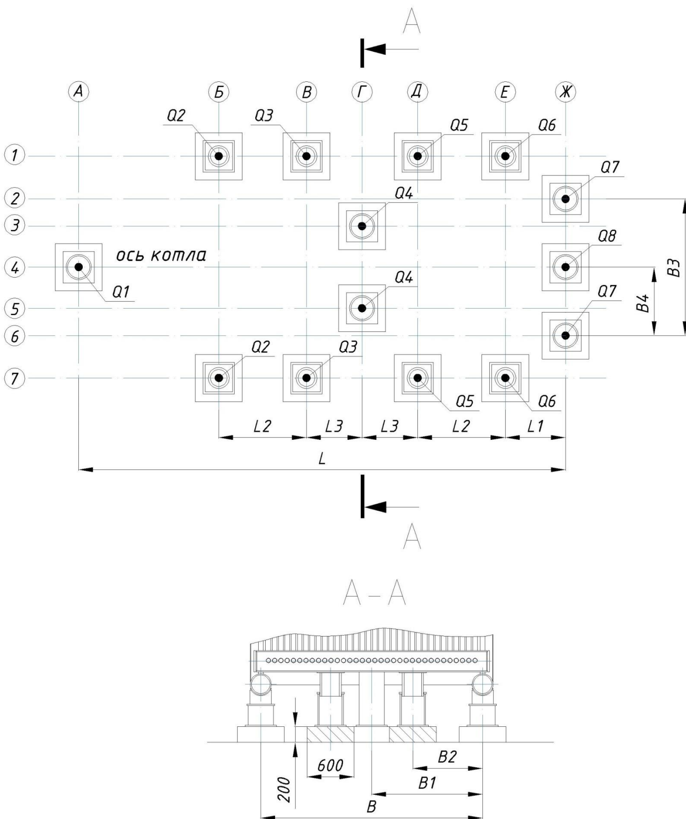
Рисунок 6 – Схематическое изображение нагрузок на фундамент
